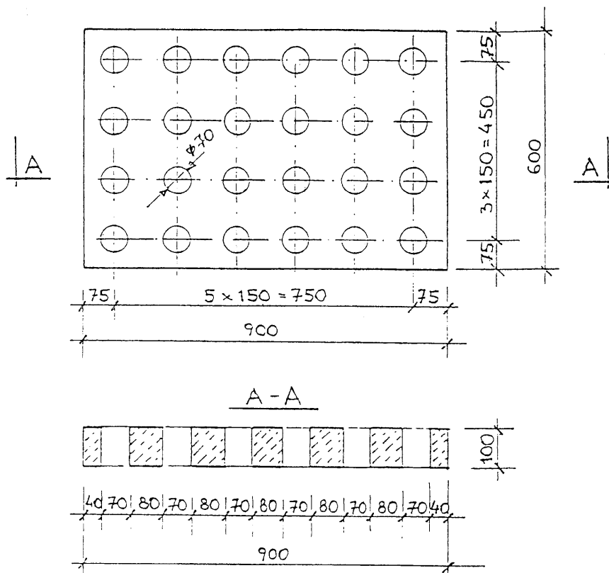
Rys. 1. Przykłady płyt betonowych
